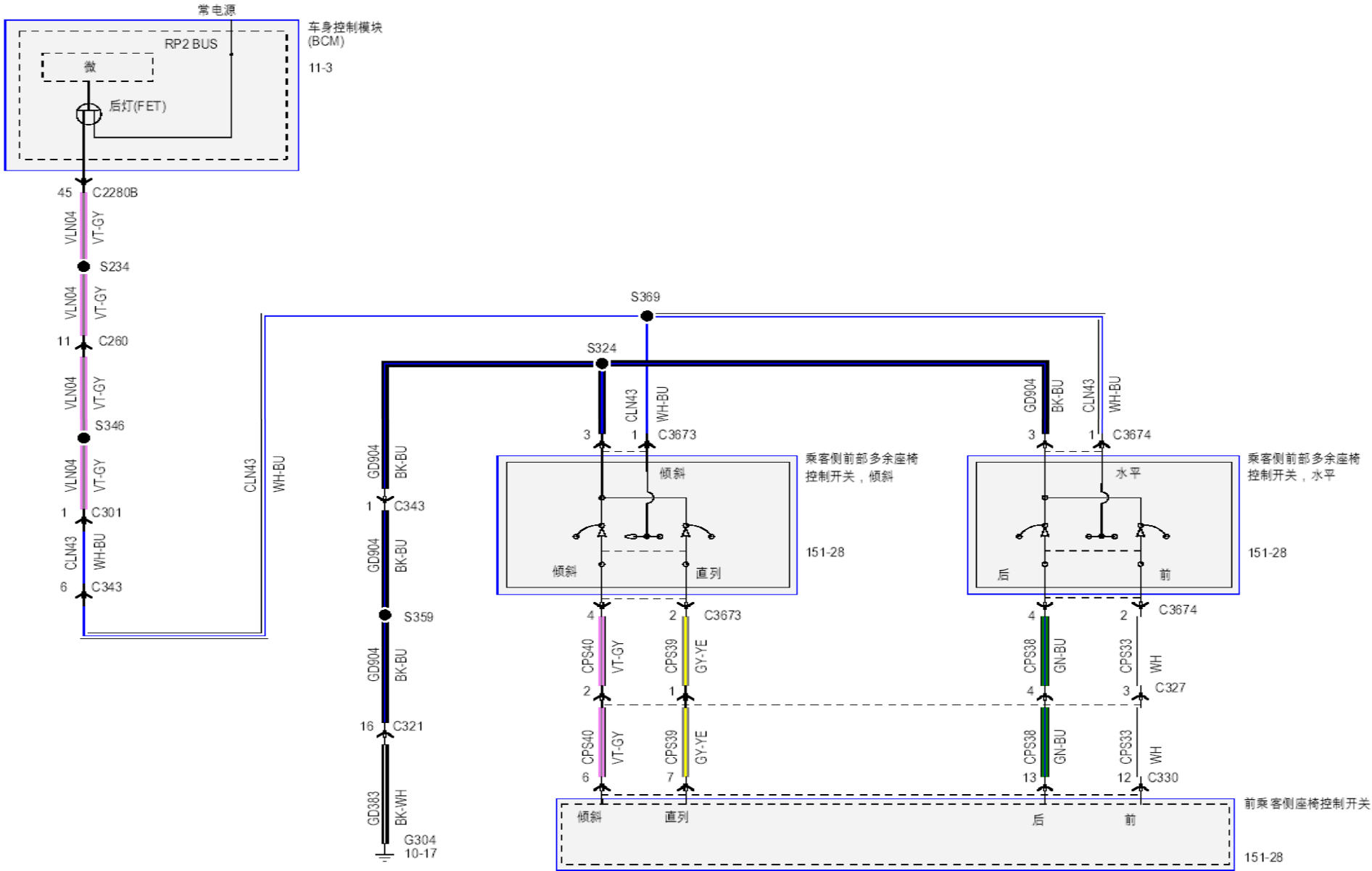
多余座位控制 - 乘客侧
